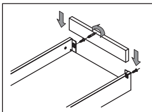
задняя стенка ящика
