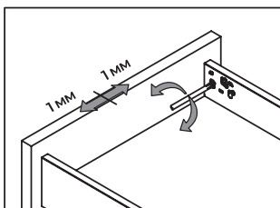
регулировка фасада вправо | влево
